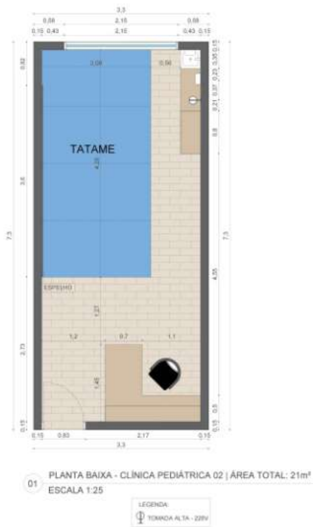
Figura 11 – Análise Dimensional CP2
